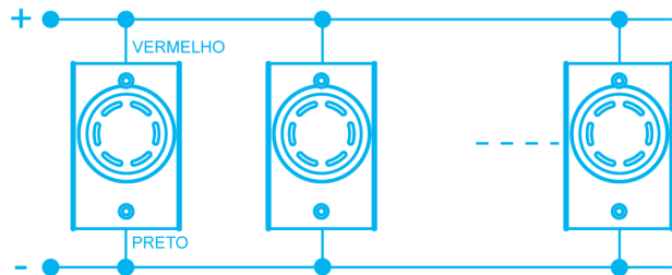
LIGAÇÃO DA SIRENE CONVENCIONAL SBC
